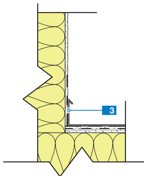
DETALJ 21MW - TYPE 2 - II
