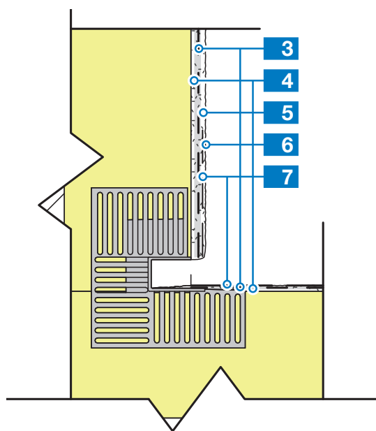
DETALJ 33MW - B2
