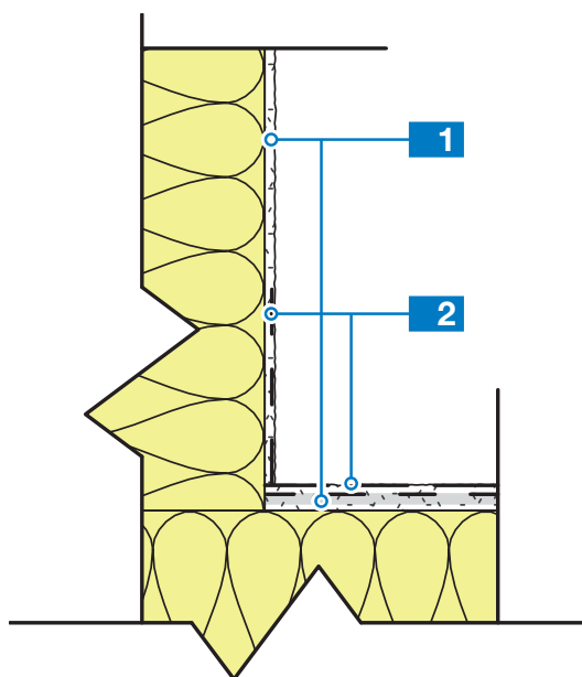
DETALJ 21MW - TYPE 2 - I
