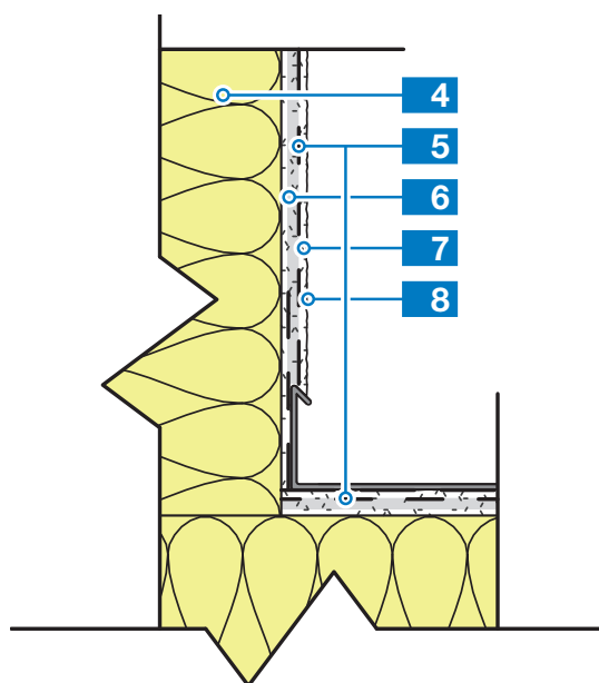
DETALJ 21MW - TYPE 2 - III
