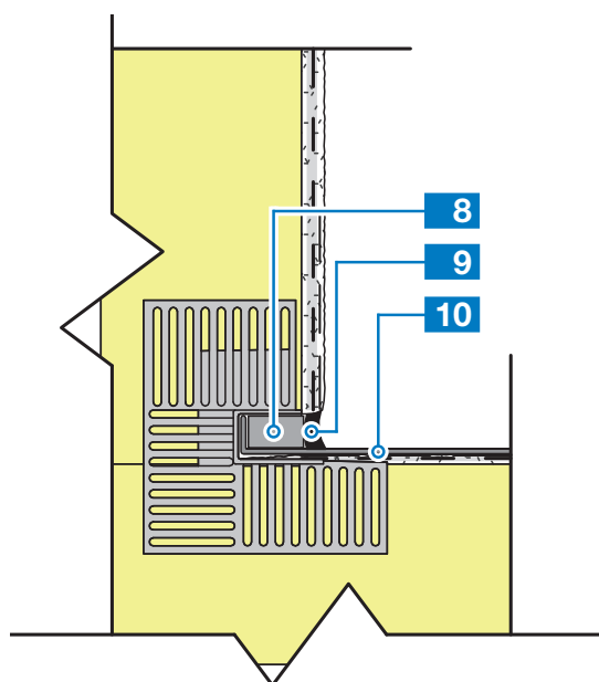
DETALJ 33MW - B3
