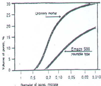
Fig. 2. Porenes kumulative volum ved EMACO S88 til støping (målt med kvikksølvporøsitetmåler) sammenlignet med vanlig mørtel med samme flyt.
